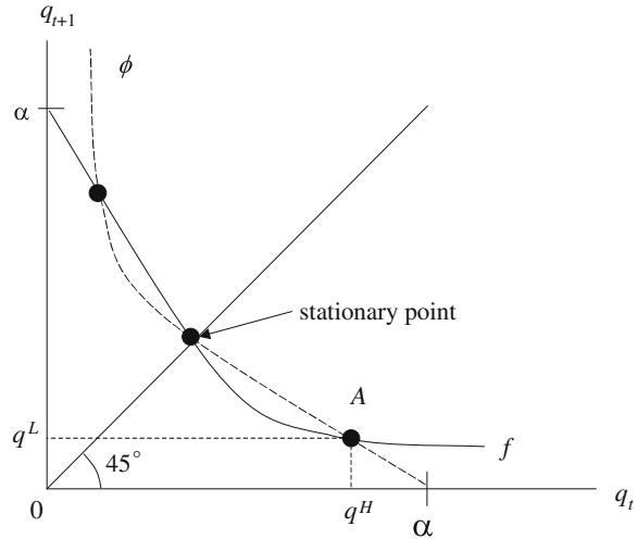
Fig. 7 A periodic equilibrium
